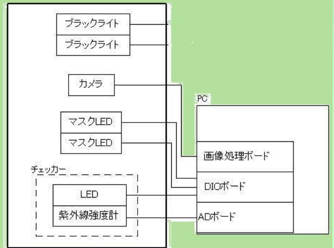
検査部(画像処理) 構成例
